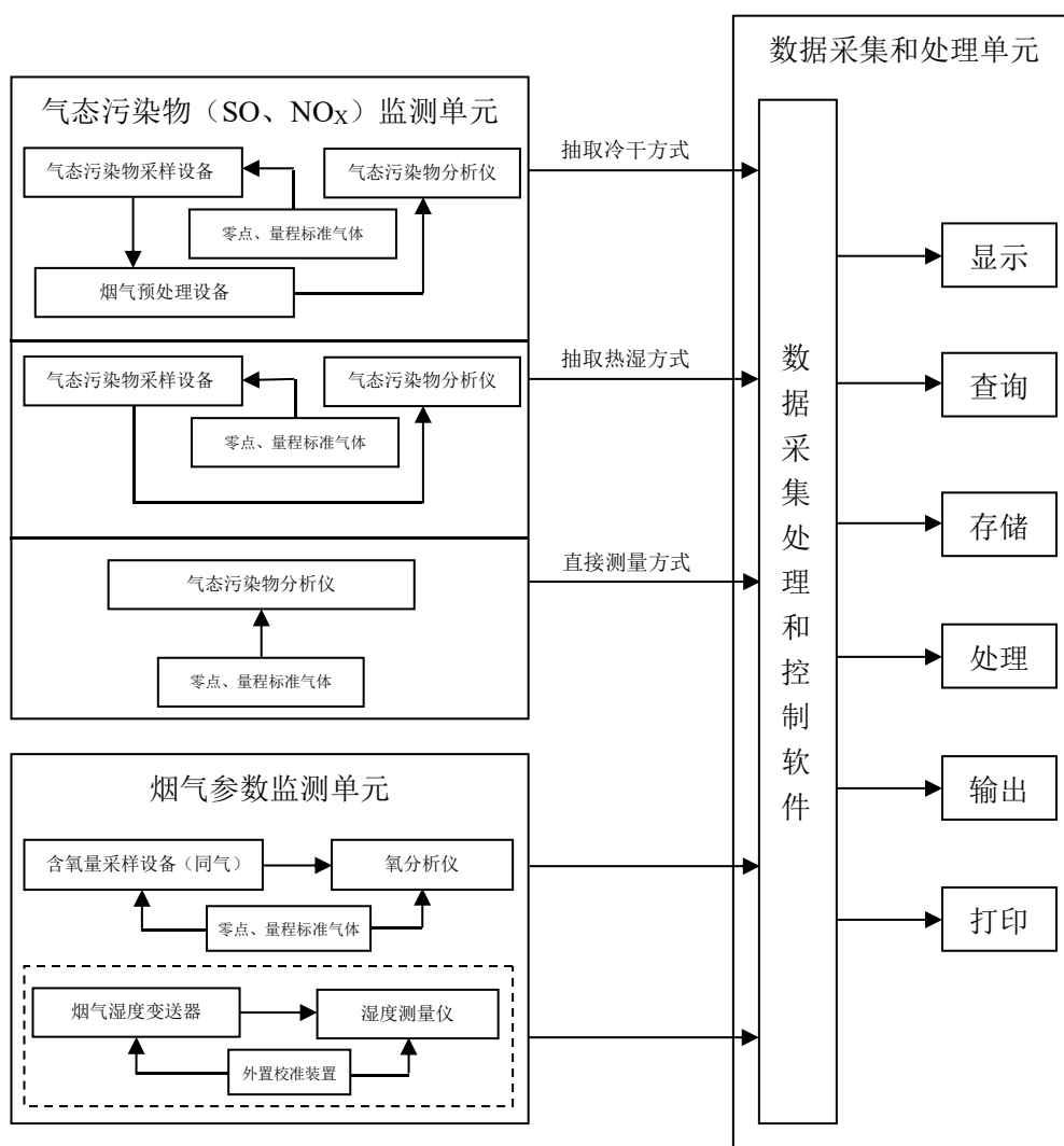
图 1 紫外吸收法便携式二氧化硫和氮氧化物测量仪器组成示意图
